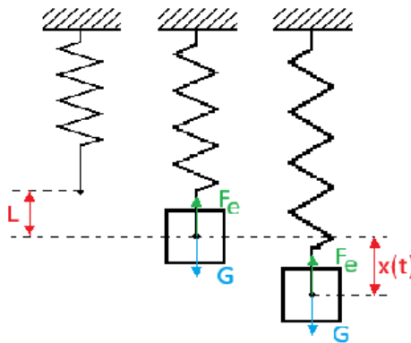
Figure 6.4: Pendulul fără frecare
