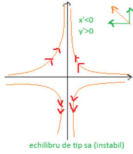
Figure 9.7: punct de echilibru de tip șa
