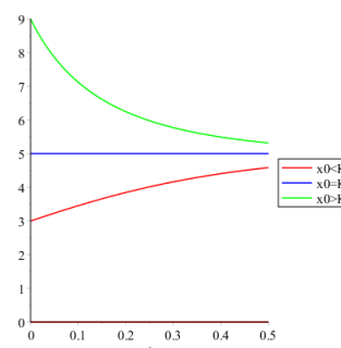
Figure 8.5: Graficul soluției ( r_0 pozitiv)
