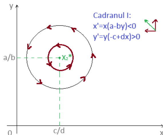
Figure 11.1: Portretul fazic centrat in X_2^*(\frac{c}{d}, \frac{a}{b}) pentru modelul (11.2)
